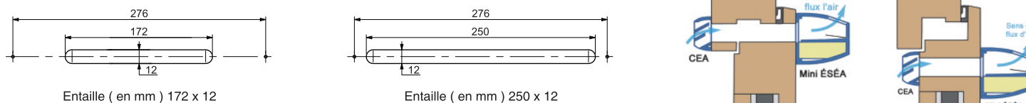
Entaille ( en mm ) 172 x 12
